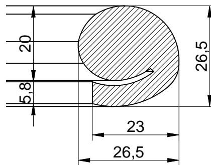
SEZIONE A-A
