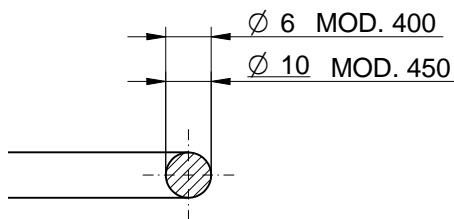
SEZIONE A-A
