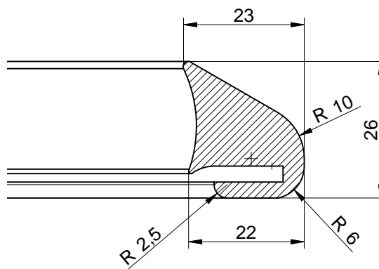
SEZIONE A-A
