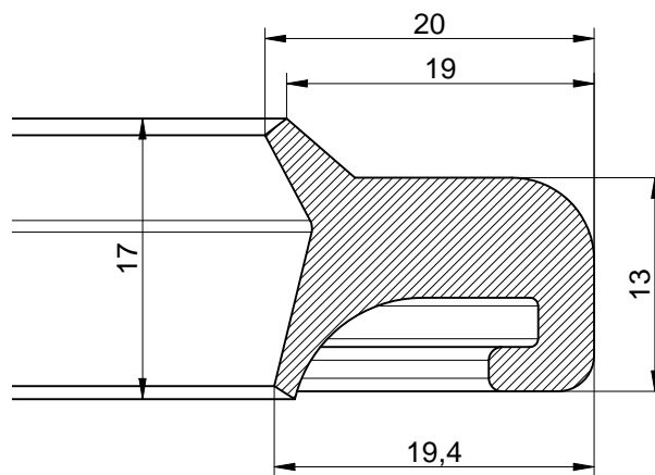
SEZIONE A-A
